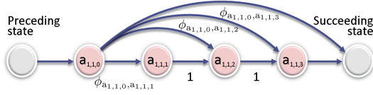
Fig. 4 状態 a_{1,1} を4つの小状態 a_{1,1,0} , a_{1,1,1} , a_{1,1,2} , a_{1,1,3} へ分割したもの. 遷移確率 \phi_{a_{1,1,0}, a_{1,1,1}} は状態 a_{1,1} が4回持続する確率に対応する.
