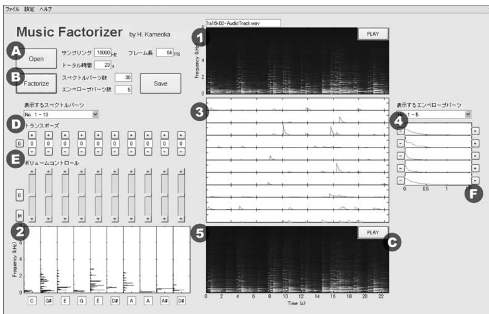
図2 MusicFactorizerの表示画面
