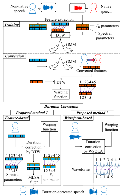
Fig. 1 提案法の処理手順
