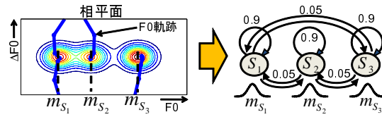
図 8 HMM の状態数の決定方法
