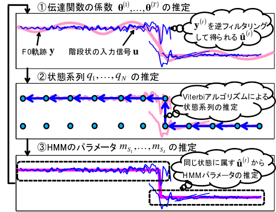
図5 パラメータ推定のイメージ図
