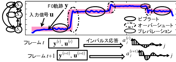
図3 時変な F0 制御モデルへの拡張
