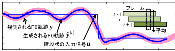
図 6 F0 軌跡の生成
