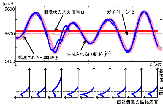
図 10 推定結果の例 1
