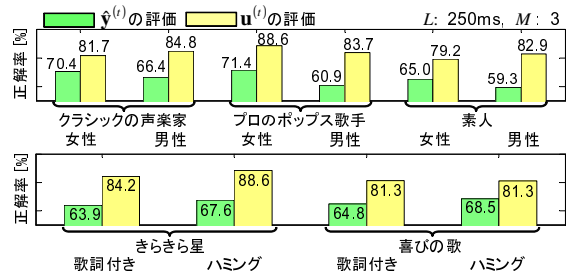
図 13 歌唱者、歌唱曲ごとの推定性能
