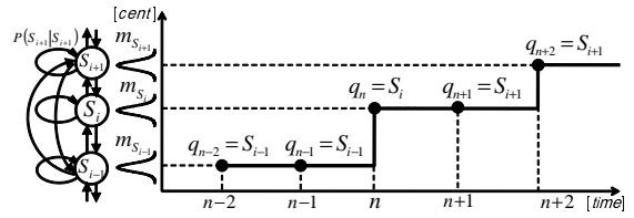
図 2 階段状の入力信号のモデル化
